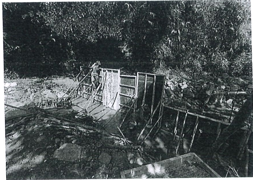
ก่อสร้างฝายคอนกรีตเสริมเหล็ก ฝายนาปลาชิว หมู่ที่ 7 บ้านชำปูน ตำบลบ้านฝาย อำเภอน้ำปาด จังหวัดอุตรดิตถ์
